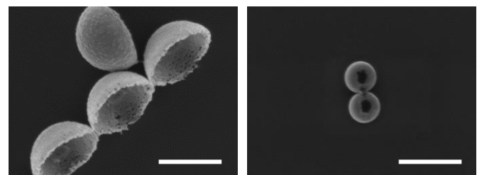
図1. 作製した金属ナノモータの電子顕微鏡写真。(左) 電子ビーム蒸着装置を用いて成膜したモータ。(右) スパッタ装置を用いて成膜したモータ。スケールバー: 500 nm。
